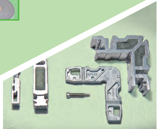
Fenstereinbauteile, Beispiele
